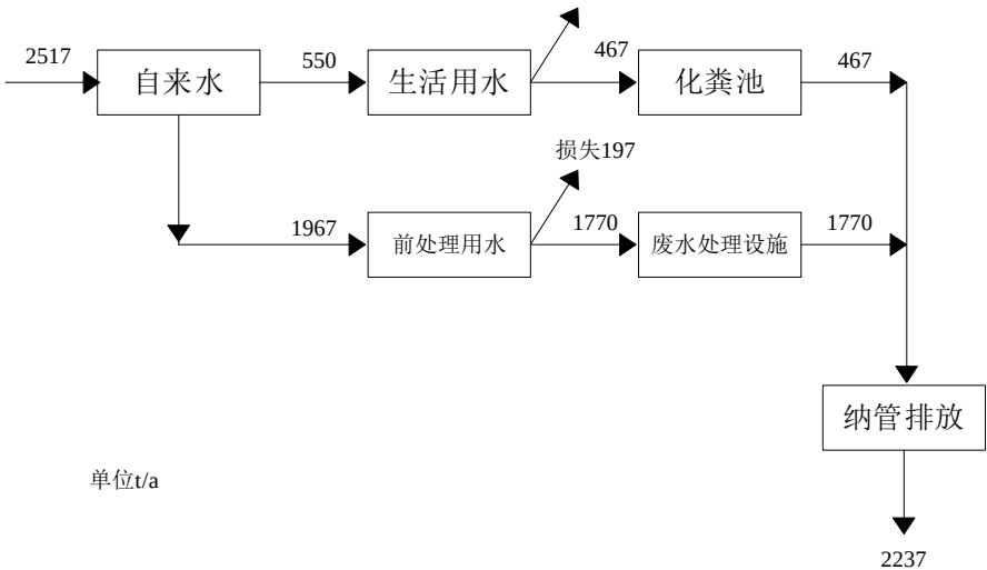
图3-3 本项目水量平衡图
